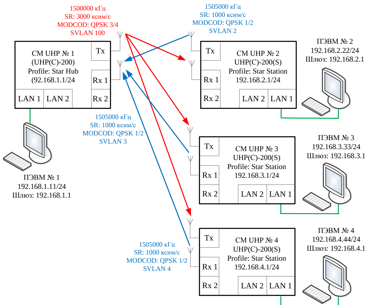
Рисунок 5. Сеть топологии «звезда» (TDM/TDMA)
