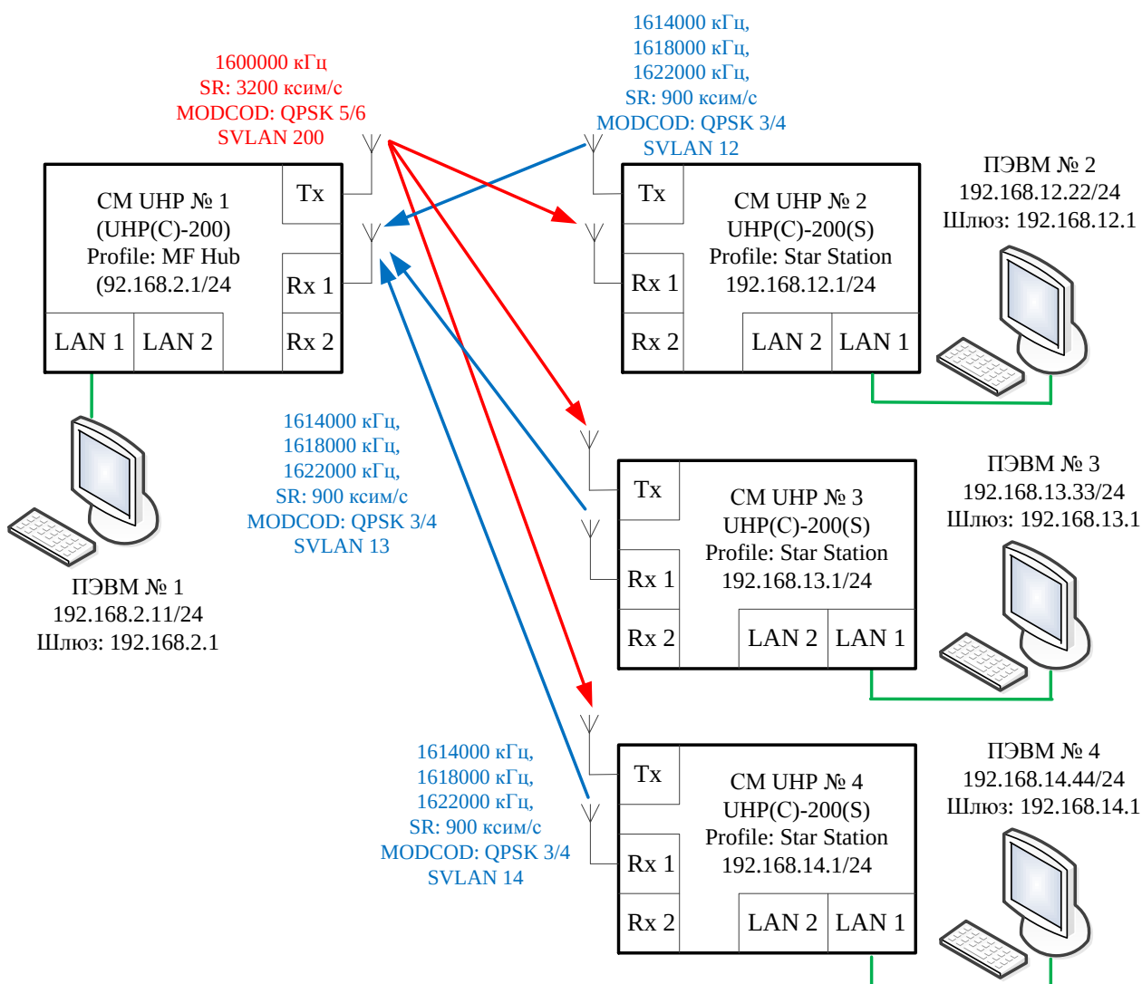
Рисунок 6. Сеть топологии «звезда» (TDM/MF-TDMA)
